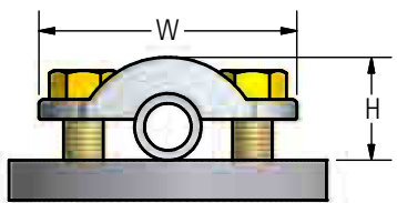
PB-AA
