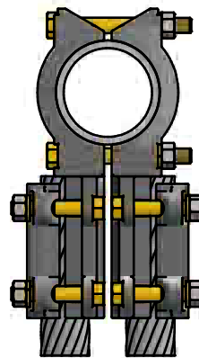
BP2CV-AA
