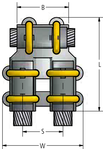
U2T-AA
